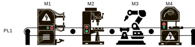
Fig. 5. Production line.
